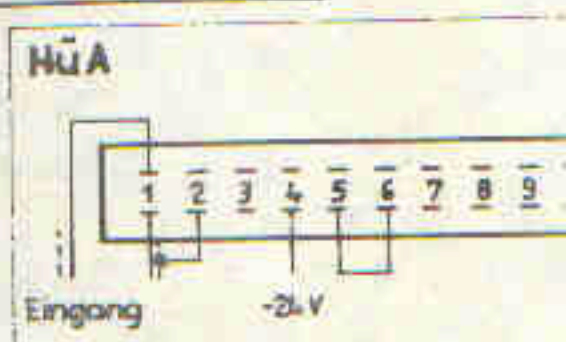
Belegung der Buchsenleiste (auf die Lötösen gesehen)
