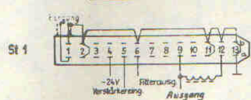
Belegung der Steckerleiste (auf die Stecker gesehen)
